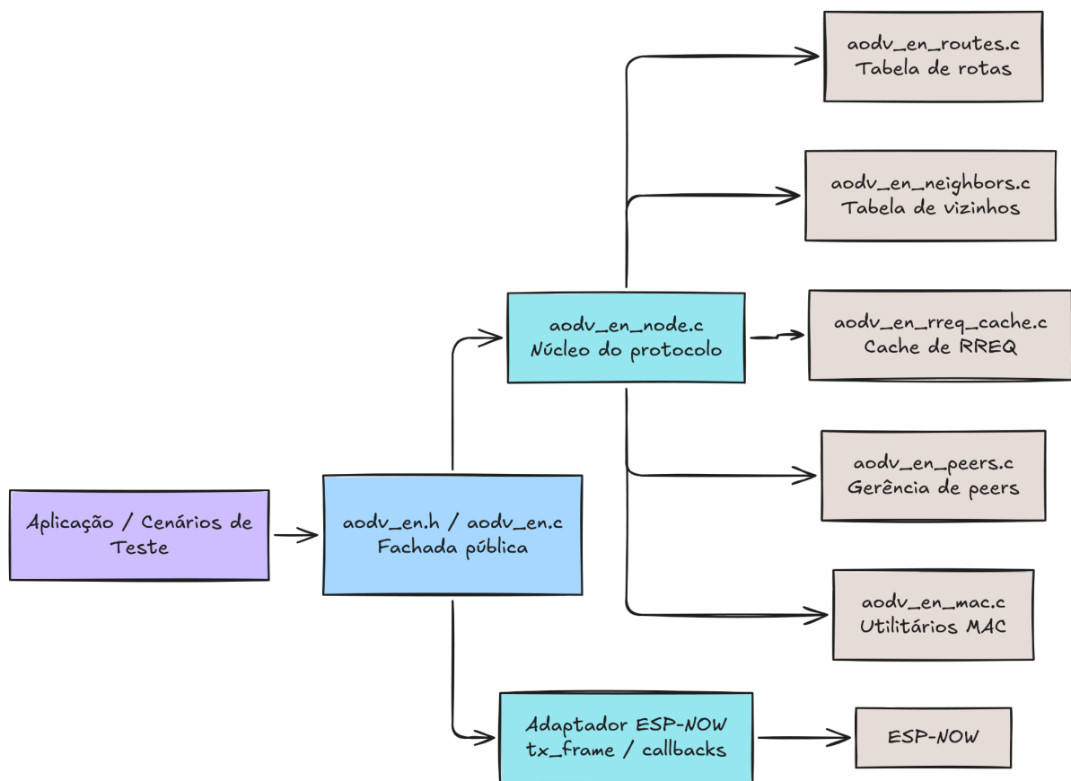
Figura 4 – Estrutura modular da implementação do AODV-EN
