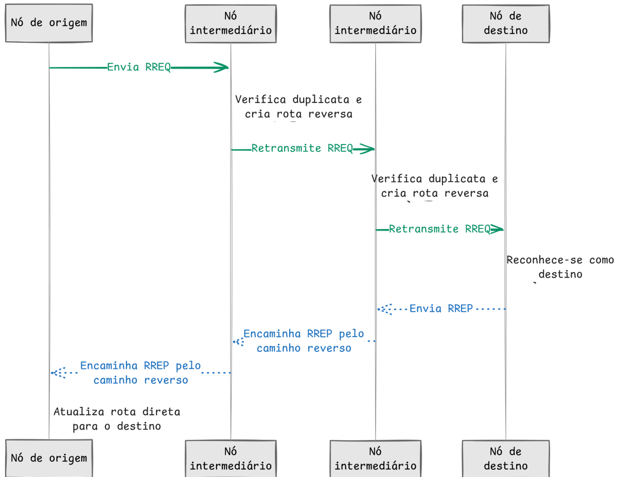
Figura 5 – Fluxo de descoberta de rotas no AODV-EN
