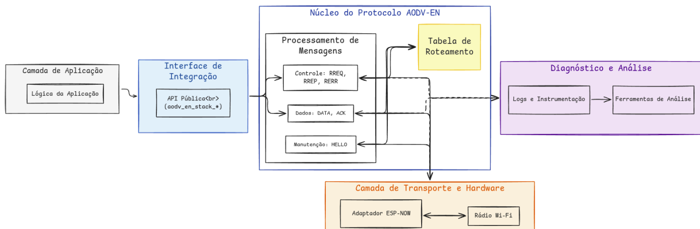
Figura 3 – Arquitetura geral do AODV-EN
